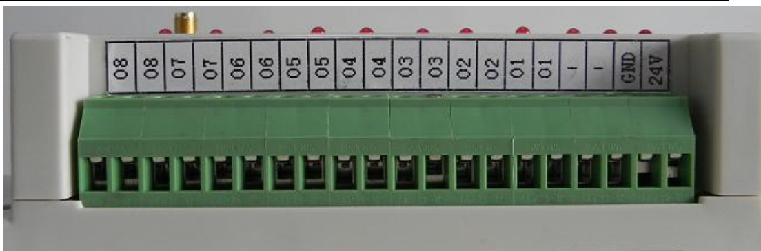
图二：COM1-开关输出及电源接线端子
