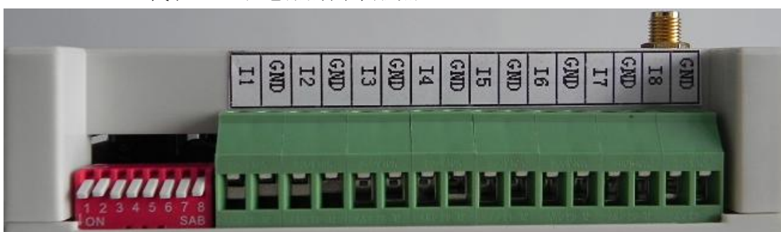
图三：COM2-开关输入端子
