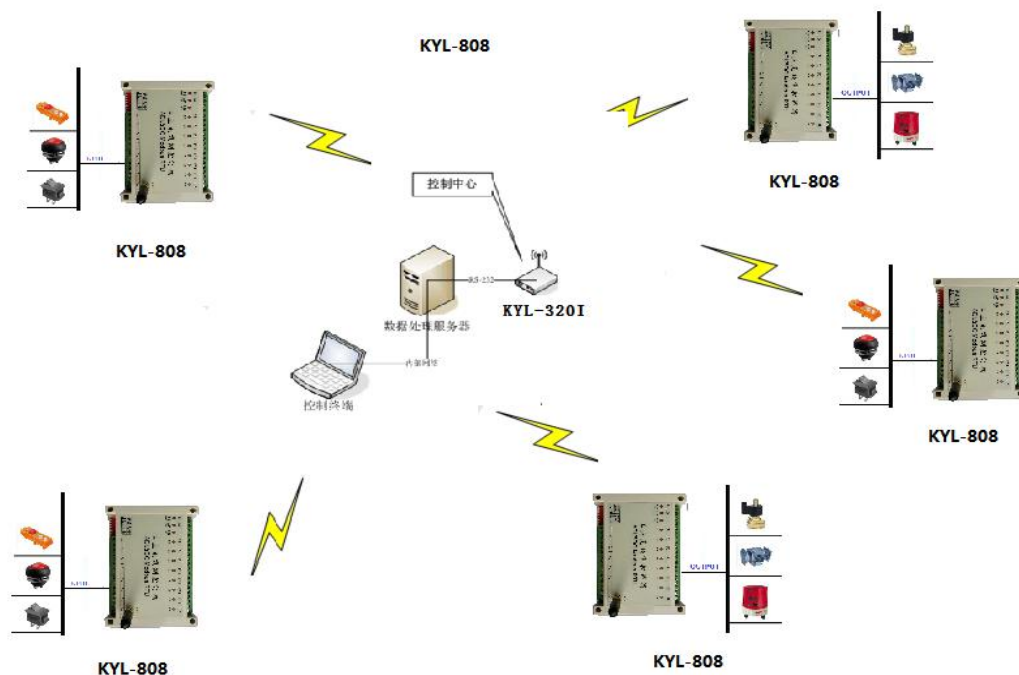
图六：采集模式组网示意图
