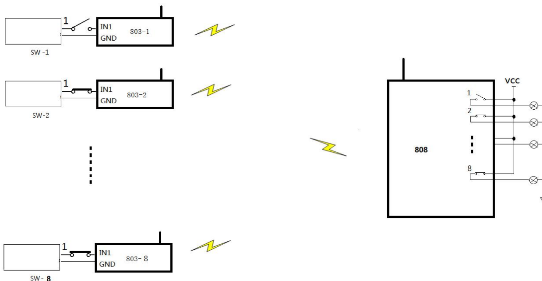
图八：8只803控制1只808
