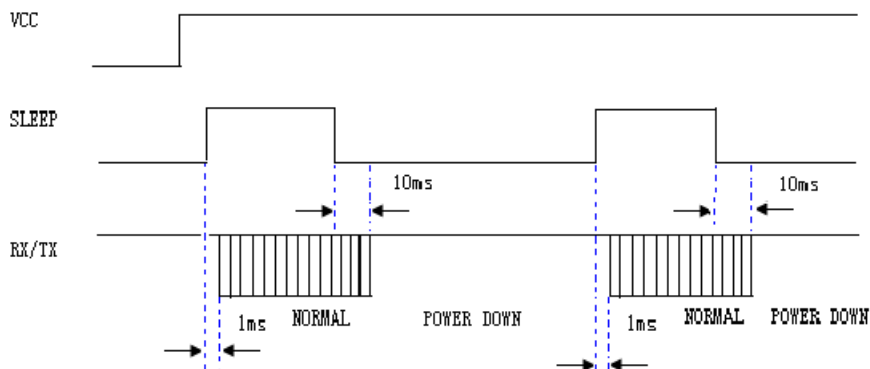
图 4：休眠时序图
