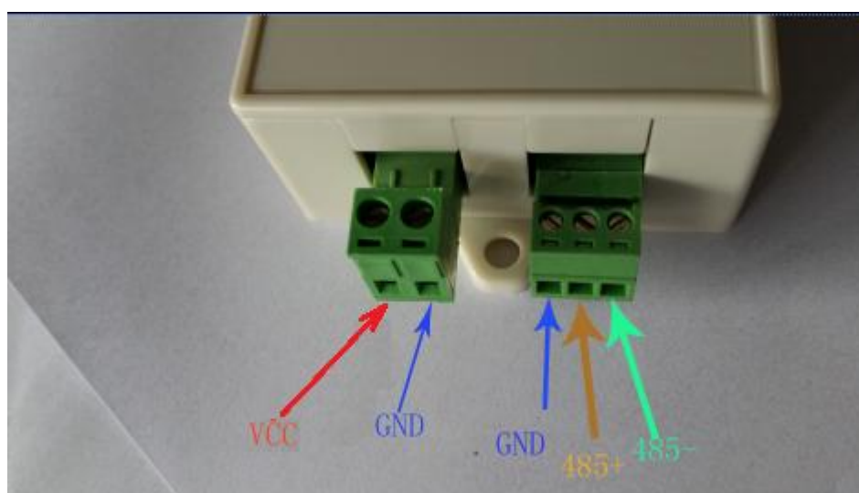
图一：接口端子
