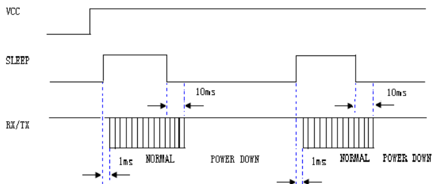
图 4：休眠时序图
